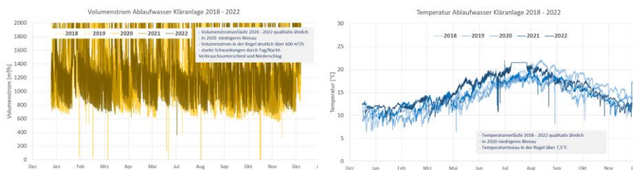
Abbildung 6: Verlauf Volumenstrom und Temperaturniveau Klärwerk
