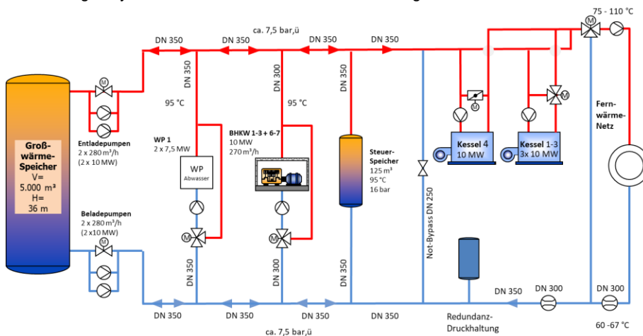
Abbildung 4: Hydraulisches Zielschema 2030
