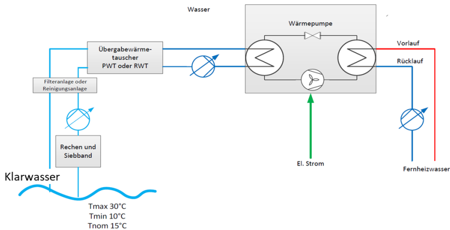
Abbildung 8: Herleitung Mindestwassertemperatur
