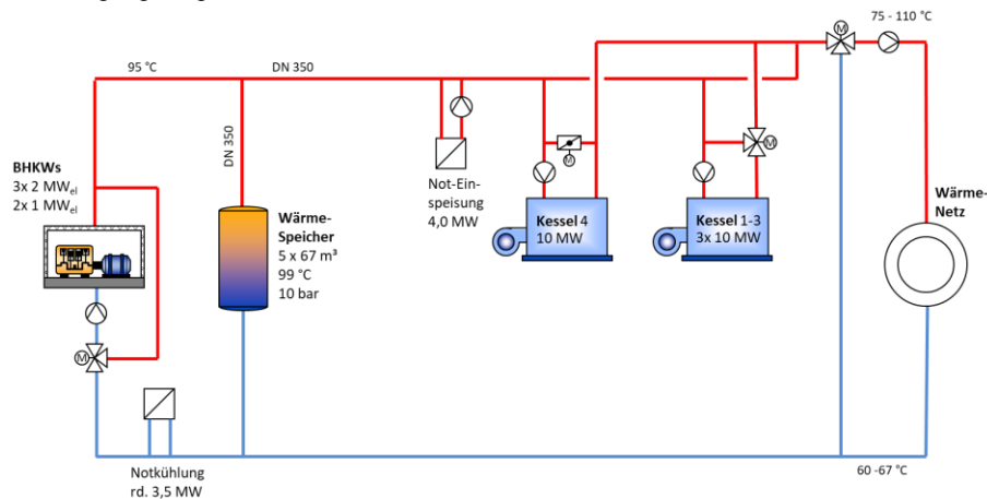
Abbildung 3: Hydraulikschema Erzeugungsstandort Hauffstraße
