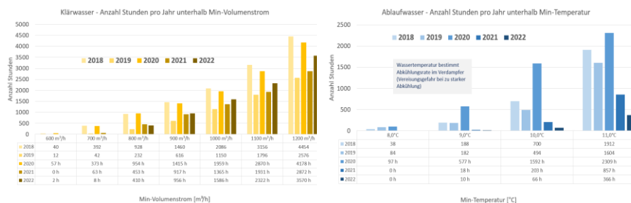
Abbildung 7: Auswertung Anzahl Stunden nach Volumenstrom und Temperaturniveau
