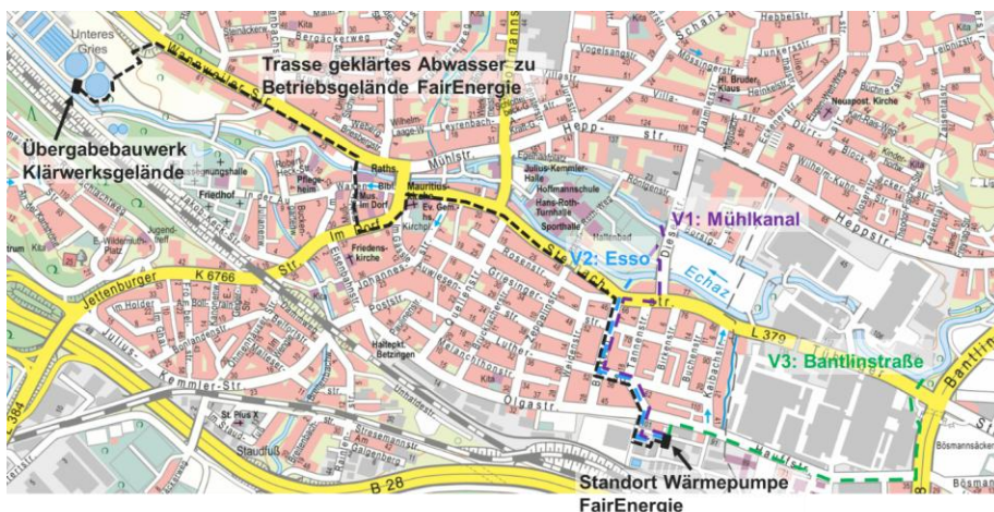
Abbildung 11: Anbindung Klärwerk zu Betriebsgelände und Einleitvarianten
