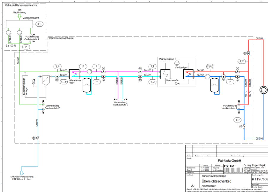
Abbildung 57: R&I-Schema der Wärmepumpenanlage
