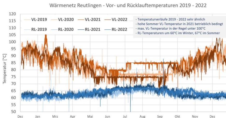
Abbildung 9: Verlauf Temperaturniveau Fernwärmenetz 2019-2022
