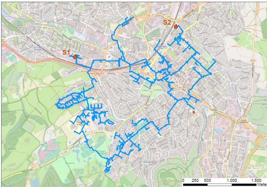
Abbildung 1: Lage des Fernwärmenetzes Reutlingen
