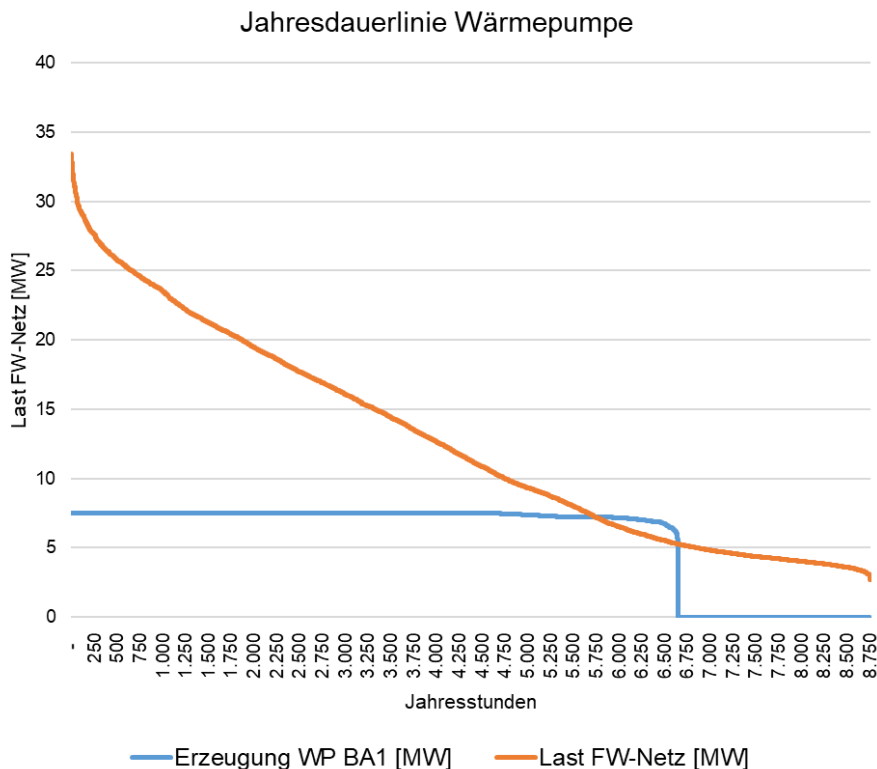
Abbildung 13: Jahresdauerlinie Wärmepumpe
