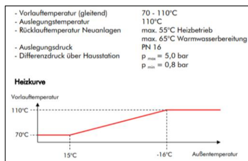
Abbildung 2: Betriebsdaten des Fernwärmenetzes Hauffstraße (Primärseite)
