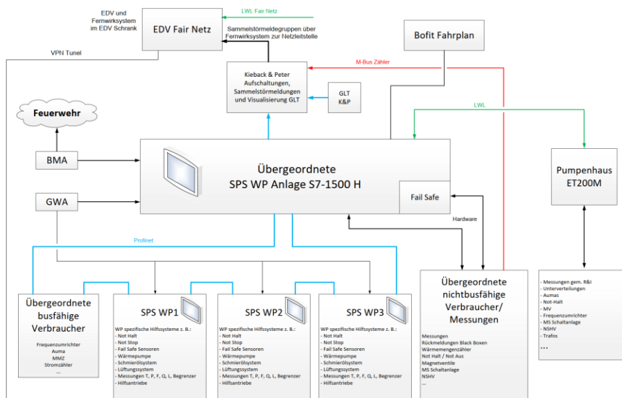
Abbildung 46: Prinzipschaltbild Leittechnik
