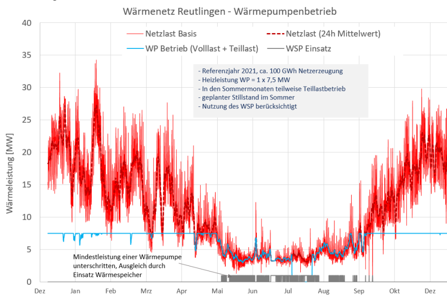
Abbildung 10: Projektion Netzlast 100 GWh
