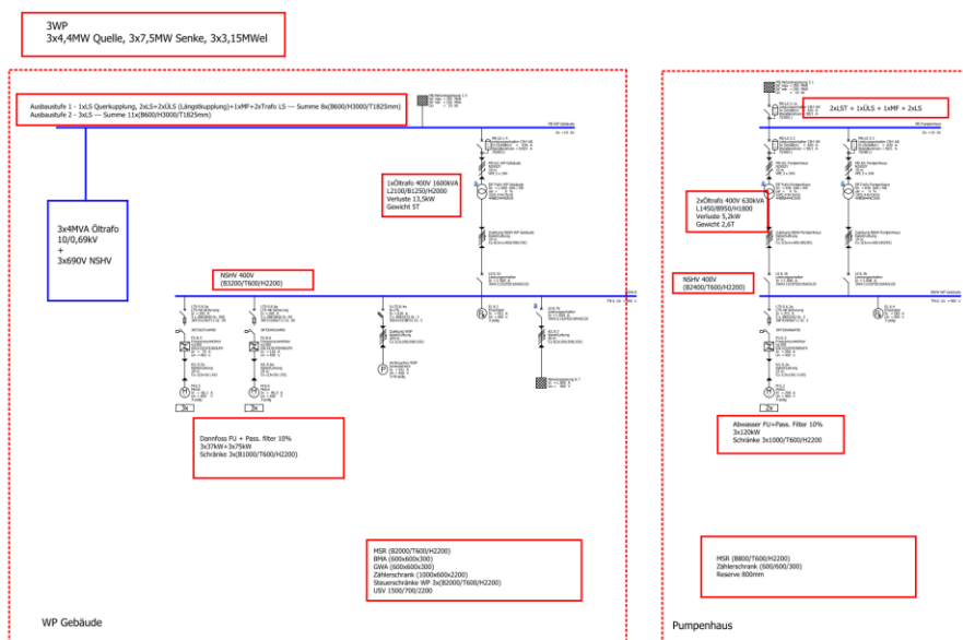
Abbildung 35: Elektrogrundschaltbild 400 V
