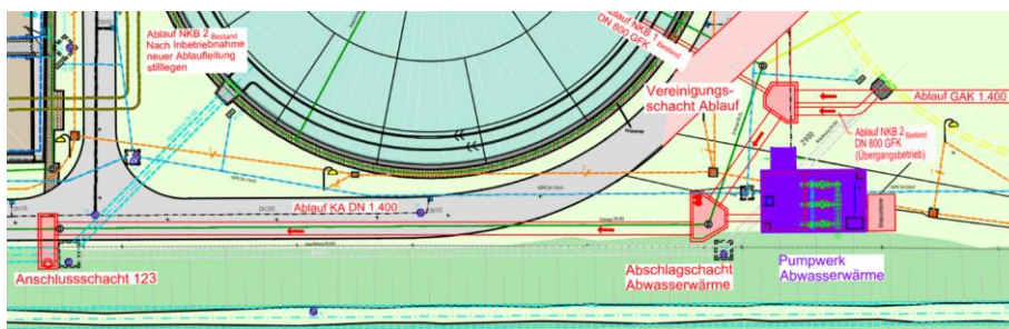
Abbildung 12: Übergabebauwerk auf dem Gelände der Kläranlage
